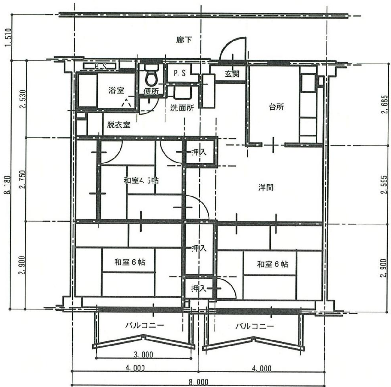
5・8号棟平面図 S=1/100
