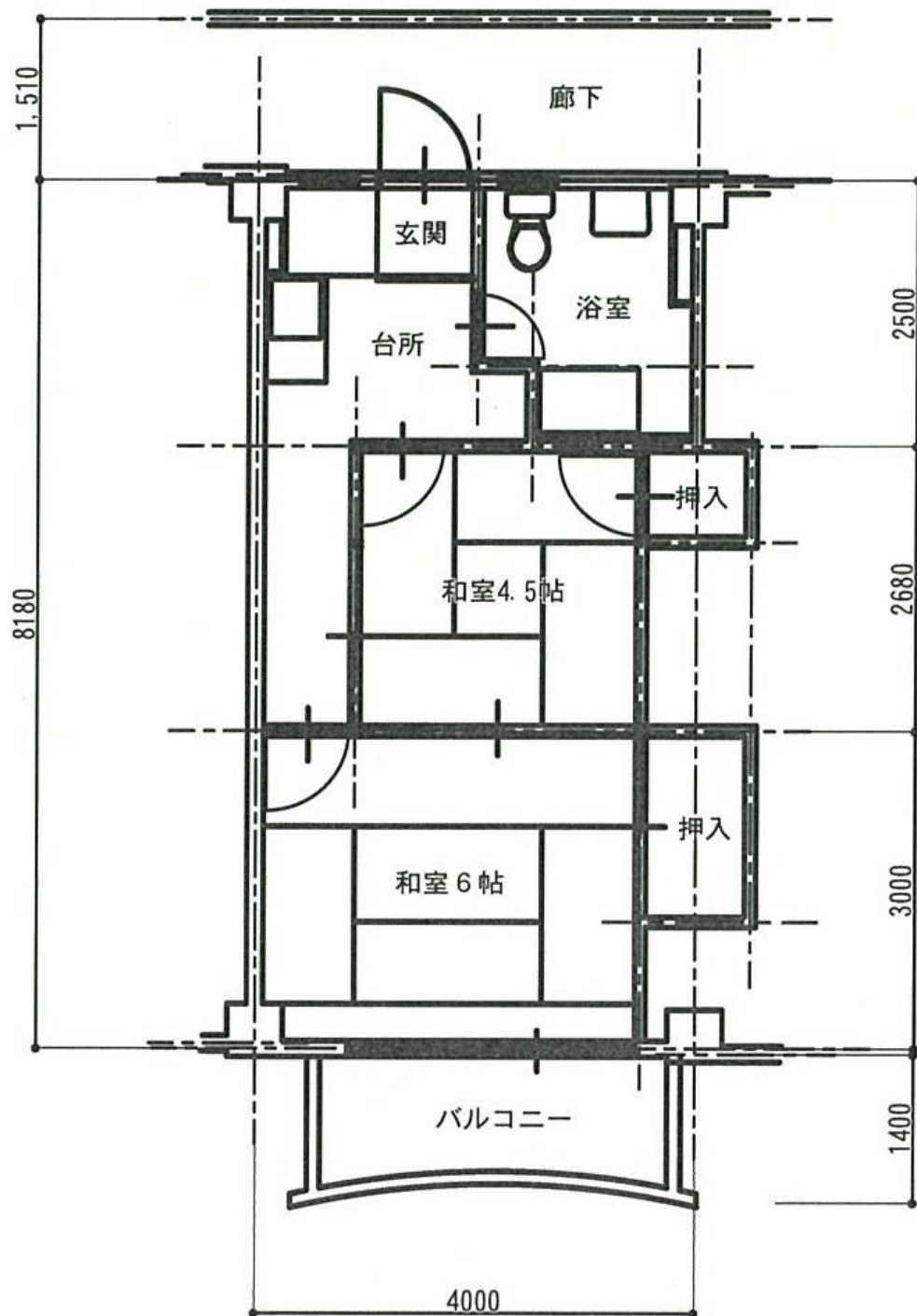
6・7号棟平面図 S=1/100
