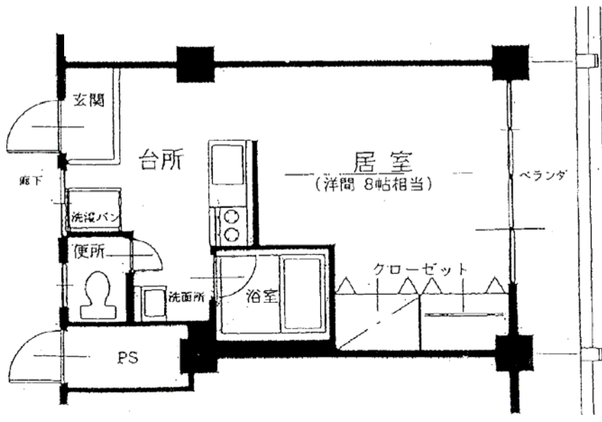
本牧単身者住宅平面図 (リニューアル室)
