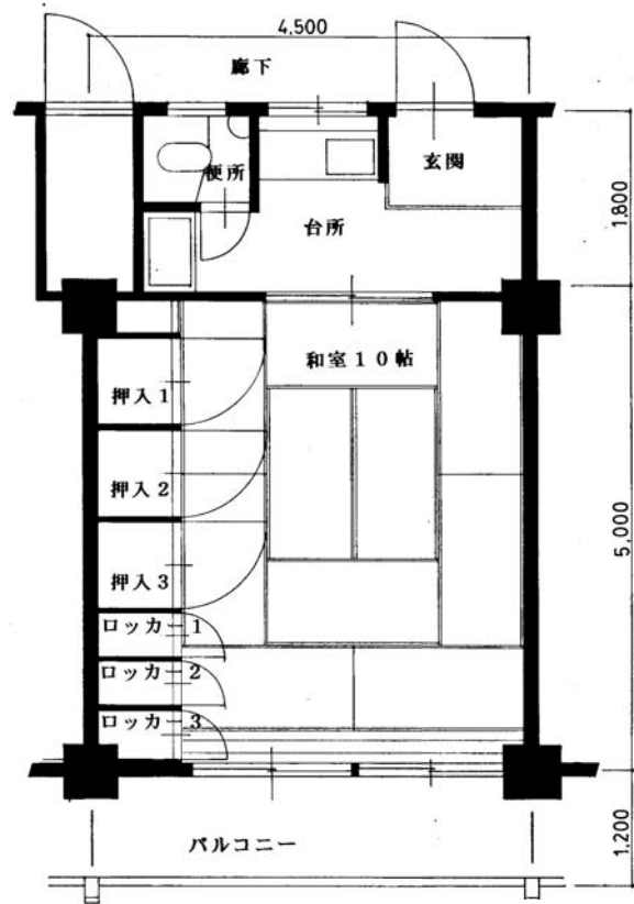
本牧単身者住宅平面図 (和室)
