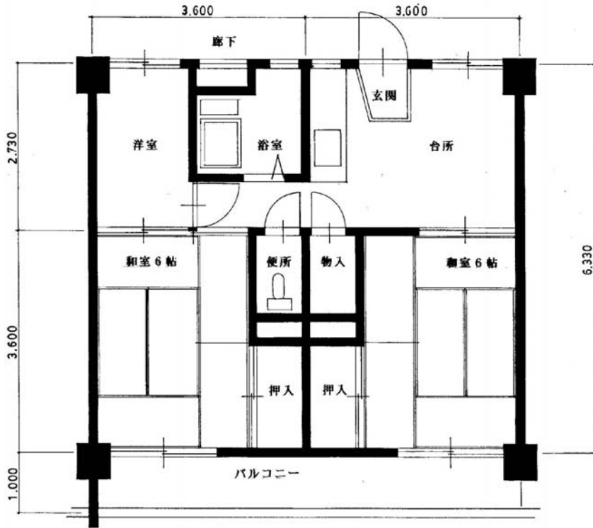
新山下 1号棟平面図
