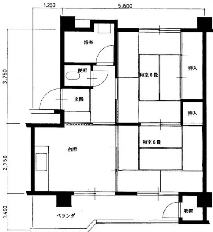
新山下 2号棟平面図
