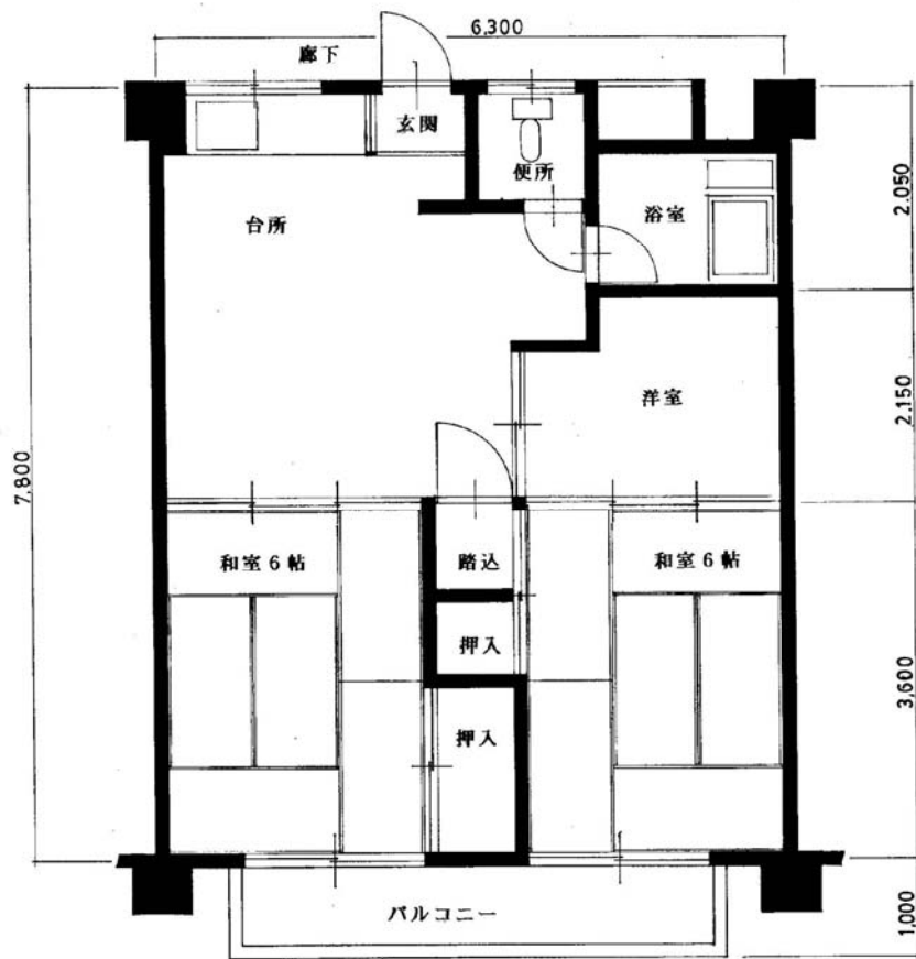
杉田PH平面図
