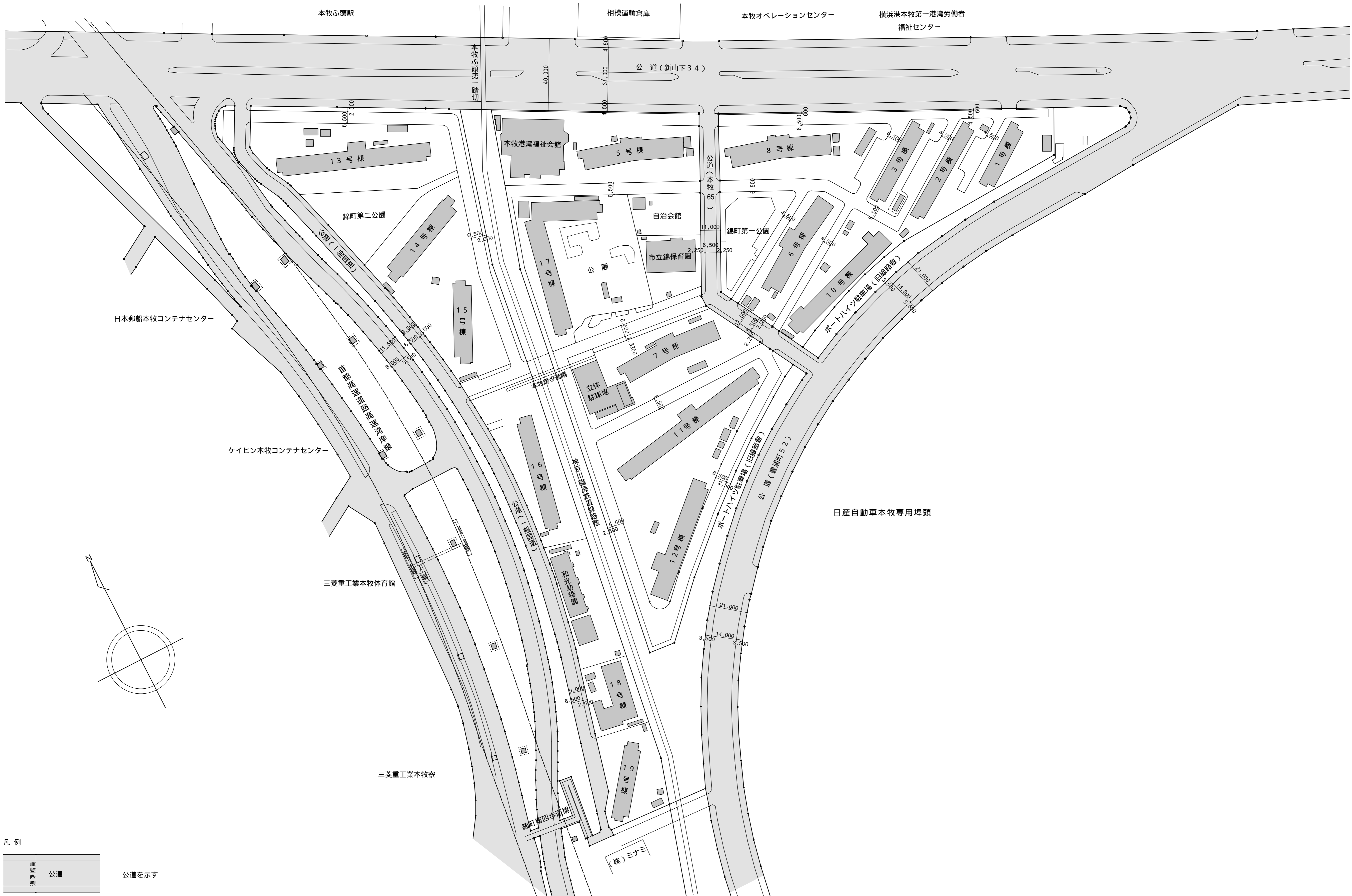
本牧ポートハイツ全体配置図 1:1,000
